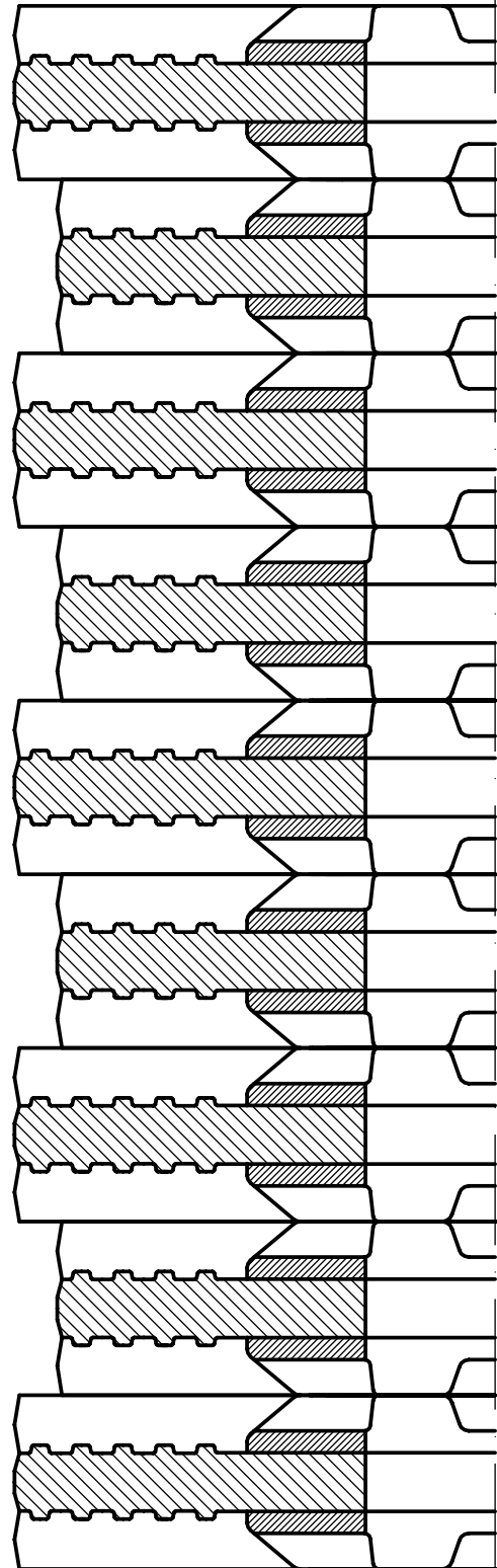
Trübezulauf feed eye
